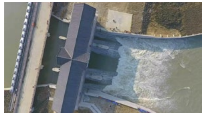
金泽水库取水闸
